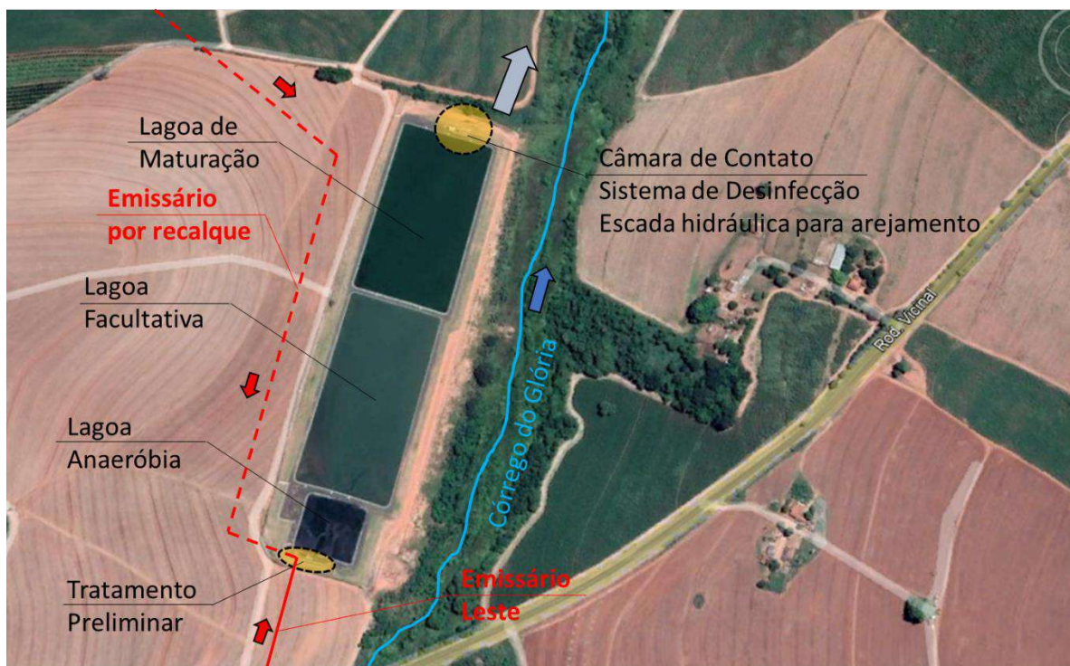
Figura 6.3 Sistema de afastamento dos esgotos e localização da ETE
