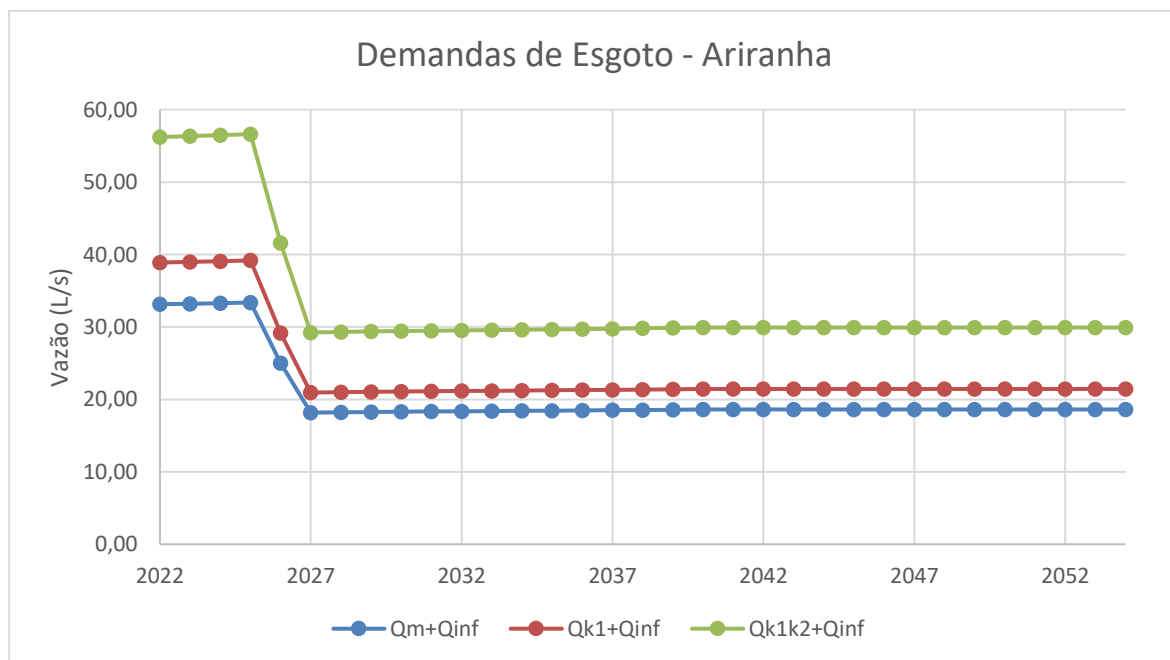
Figura 4.2 Evolução das demandas de esgoto prevista para Ariranha
