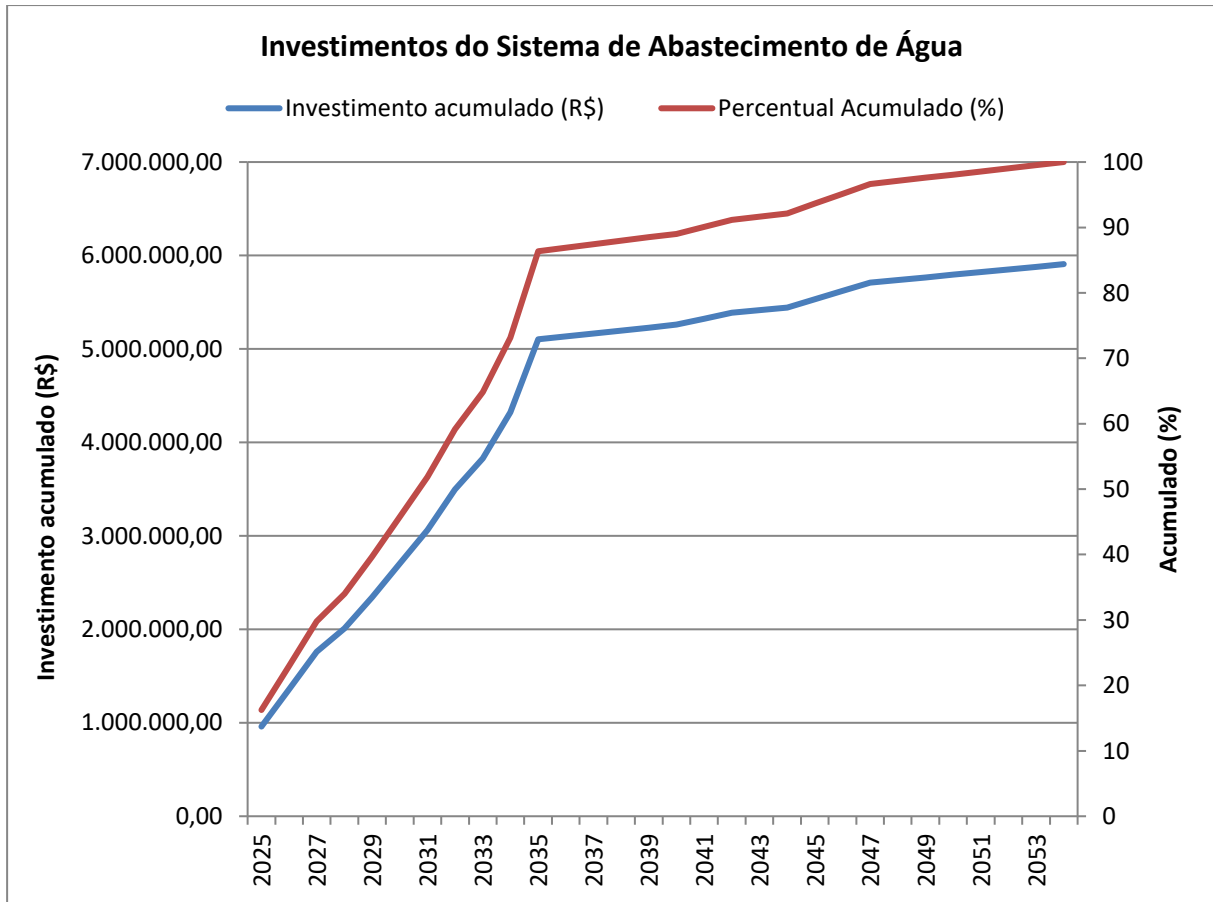
Figura 9.1 Evolução dos investimentos no Sistema de Abastecimento de Água
