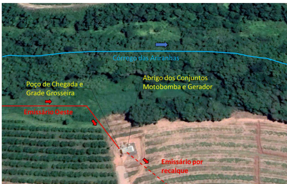
Figura 6.1 Imagem de satélite da estação elevatória de chegada do emissário oeste
