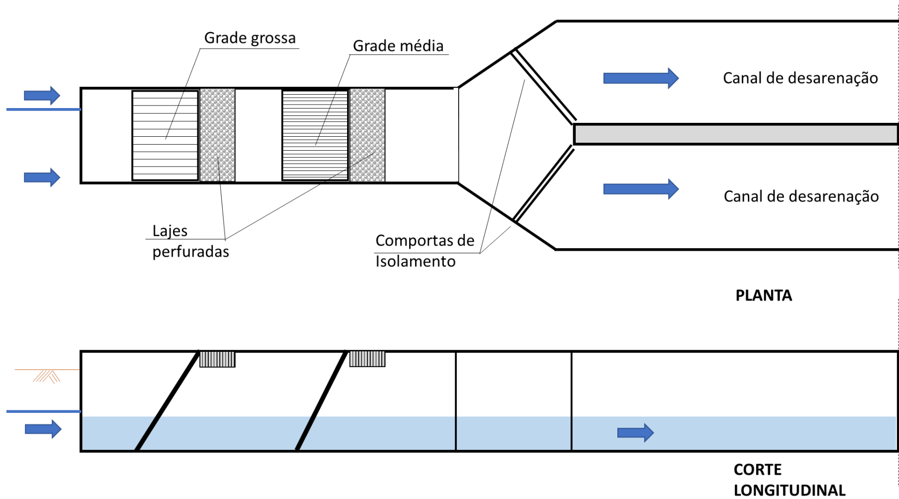
Figura 8.2 Grades de limpeza manual propostas para a ETE
