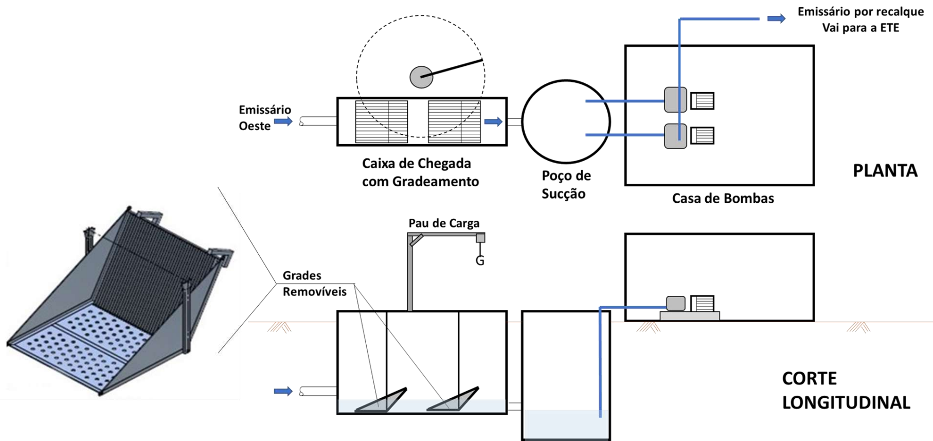
Figura 8.1 Novo sistema de gradeamento proposto
